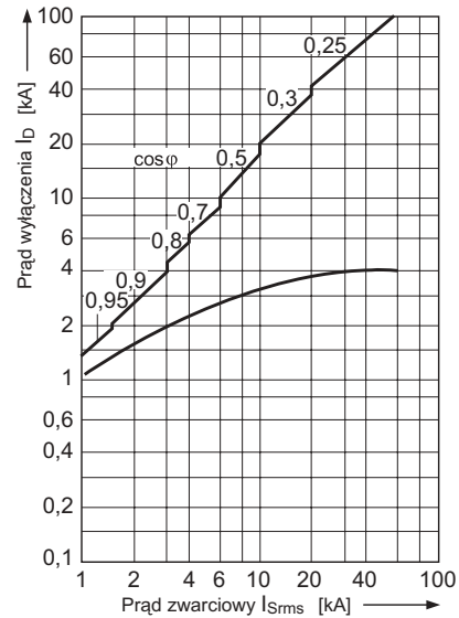
Charakterystyka ograniczenia natężenia prądu dla RMSI63-25
